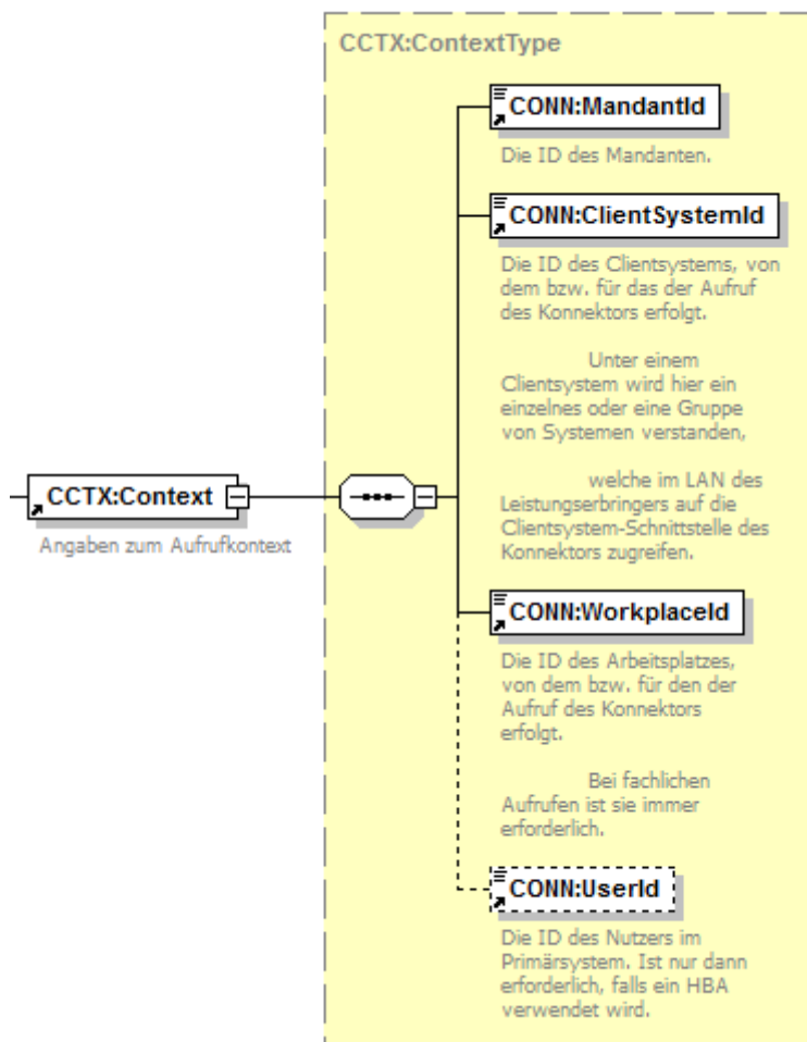
Abbildung 12: ILF_ePA_Element_Context
