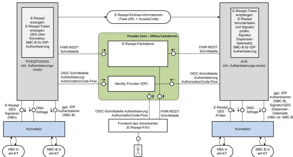
Abbildung 1: Übersicht E-Rezept-Komponenten
